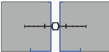
Deformatsioonivuugi ääreprofiilid
